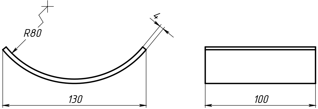
Поз.3 (Ложемент)
